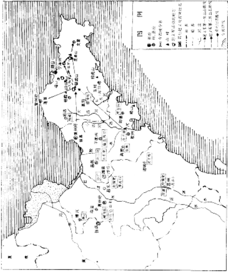
清初鲁东三南区别及第一次起义形势图
