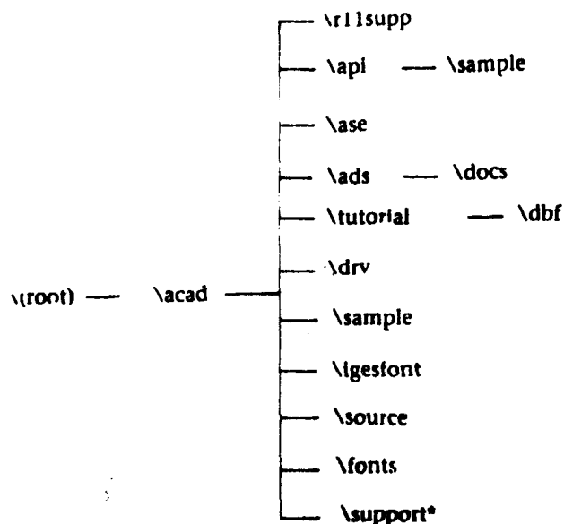
图 1-1 安装所有文件时的缺省目录结构
