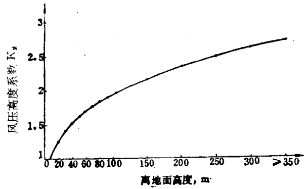
图 6.2-1 风压高度系数
