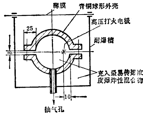
图 6.2-2 测定 \delta_{\max} 的标准试验条件
