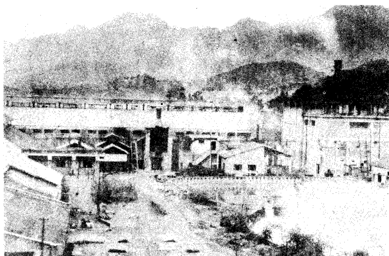
第二十四工厂主要生产车间,右:动力部, 1500千瓦 发电所,中:电炉炼钢部,左:第一轧钢部。
