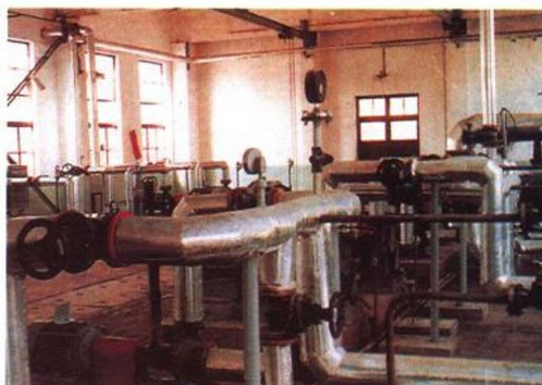
车间一角
