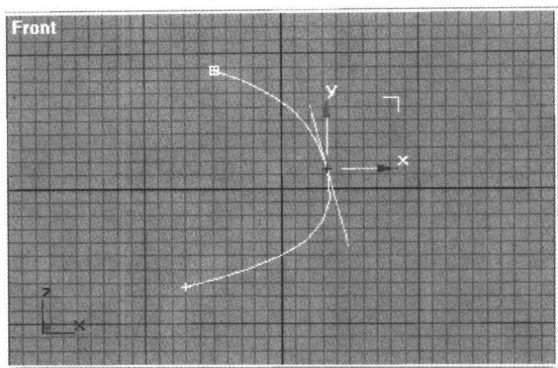
图 1-6 贝塞尔节点
