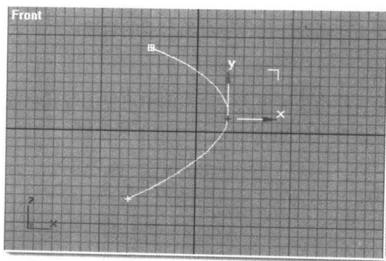
图 1-4 光滑节点
