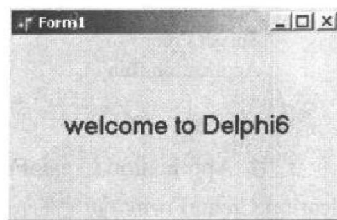
图 1-2 主窗体
