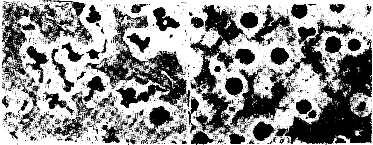
图 1-3 铸铁的两种不同组织, \times 250
