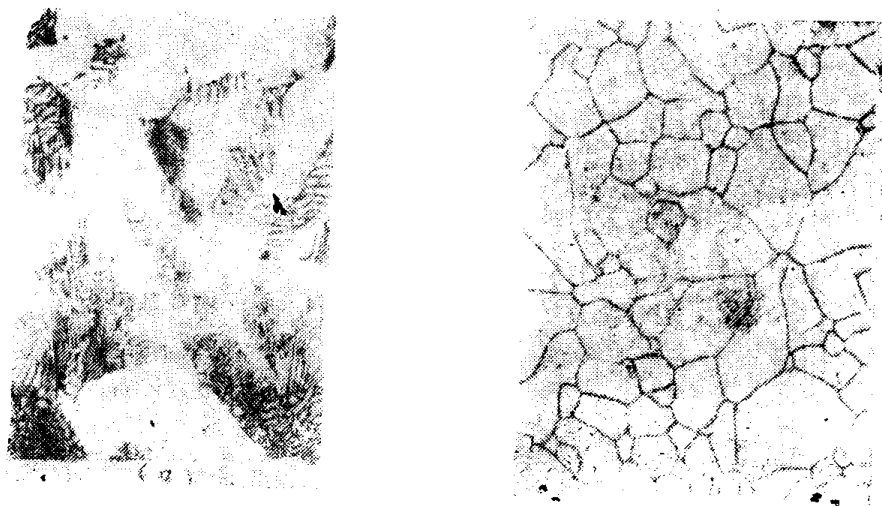
图 1-2 含碳量为0.35%的钢（ a ）， \times 450 缩1/3和纯铁（ b ）， \times 250 的显微组织
