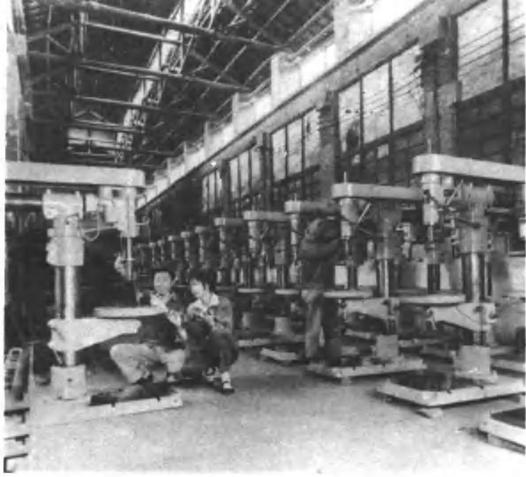
县办五小工业生产机具，装备社队 农机修配站。这是县农机修造厂生产的 立式台钻，工人正在检验，准备出厂。
