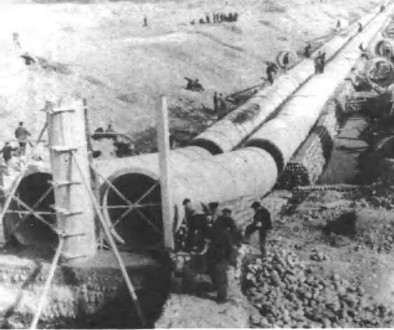
鸭子河倒虹管工程。
