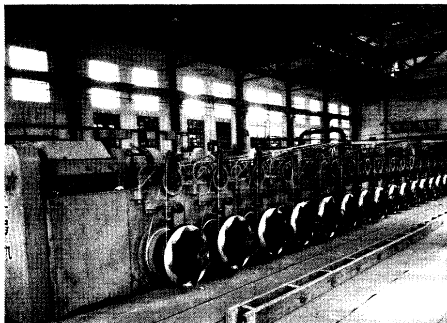
天津市大成五金厂自动化热镀锌生产线
