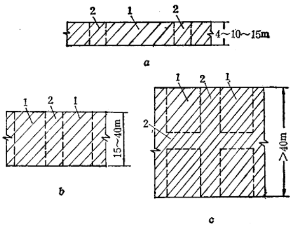
图 1-2 矿块的布置方式
