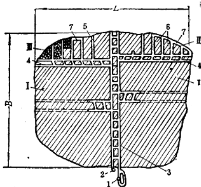
图 2-3 盘区和采区的划分
