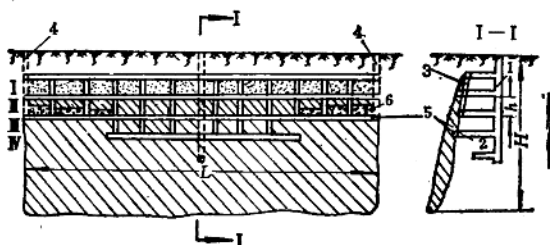
图 2-2 阶段和矿块的划分
