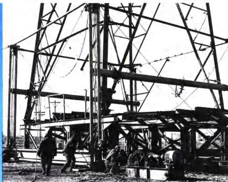
采用“开森堡”法安装井架
