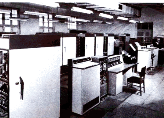
10 被中共中央国务院中央军委誉为“功勋机”的DJS-8(320机)
