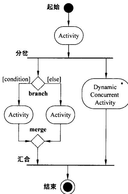
活动图
