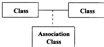
关联类
