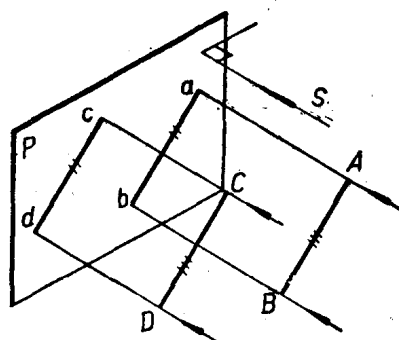
图 1-8 互相平行的两直线的投影
