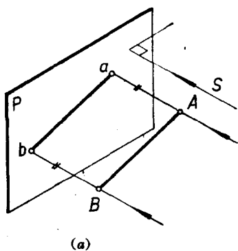
图 1-9 投影的真实性
