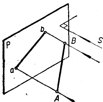
图 1-6 直线的投影
