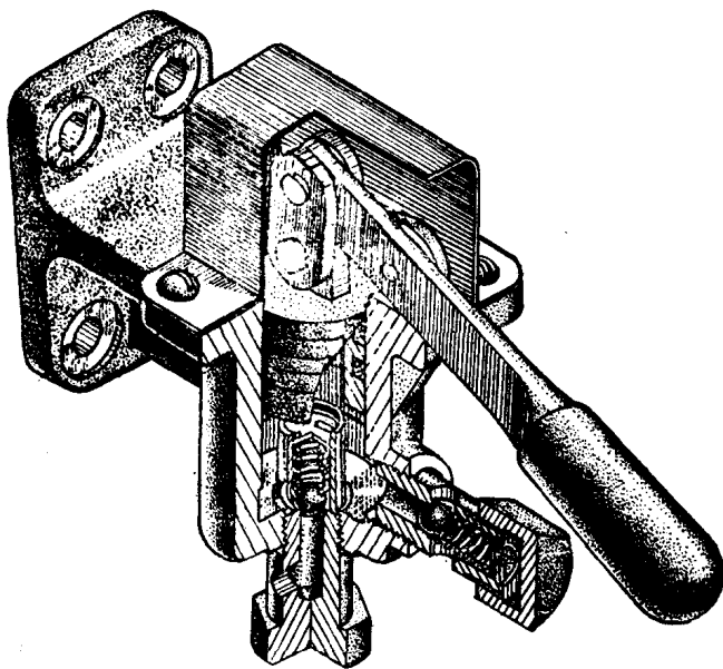
图 I 手压滑油泵的立体图
