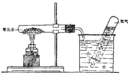
图 1-1 氧化汞的分解实验
