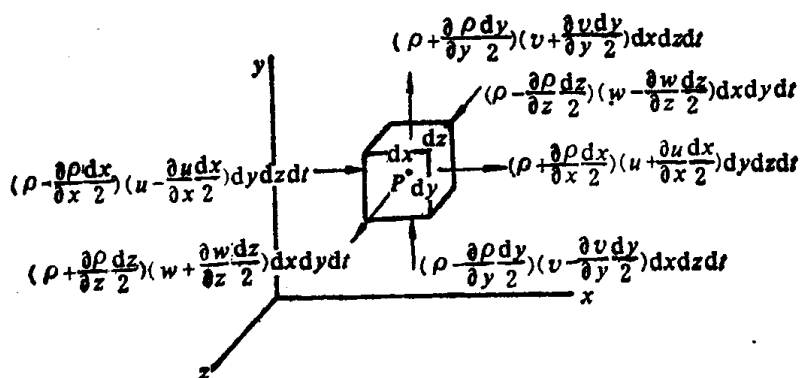
图1-3 连续方程的推导说明
