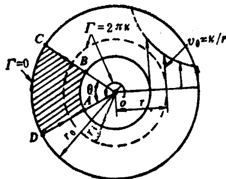
图1-1 自由涡流动
