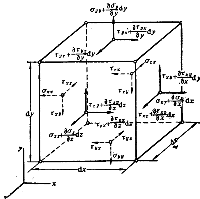
图1-2 微元流体的表面应力
