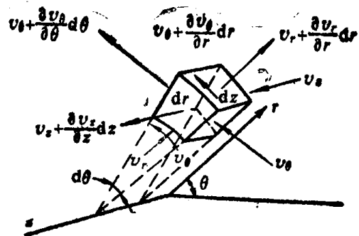
图1-4 圆柱坐标的速度变化
