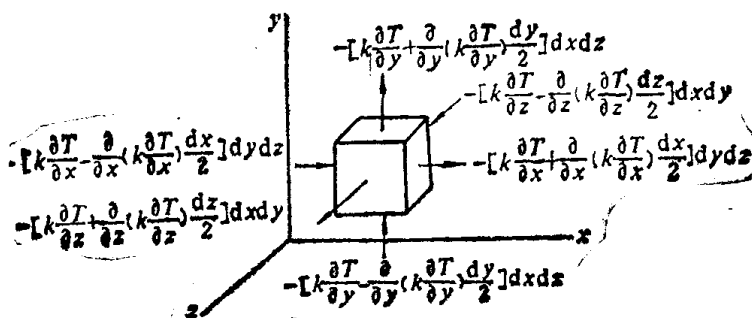
图1-5 微元质量流体的传热
