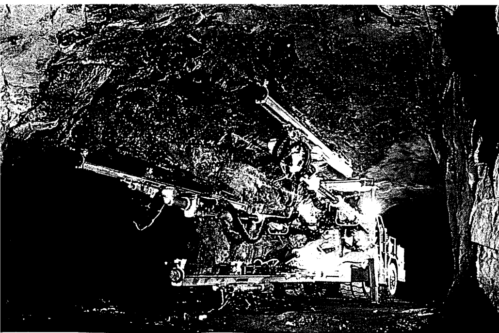
阿特拉斯·科普克公司生产的凿岩台车正在巷道中开挖。
