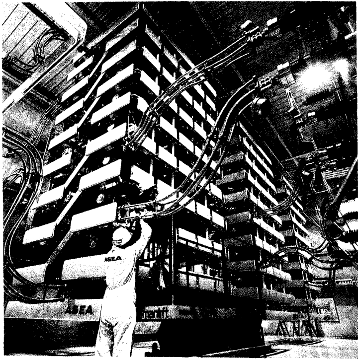
ABB公司生产的高压直流输电设备。
