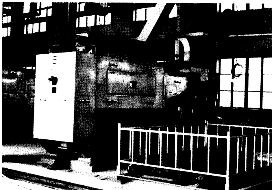
新型榨油机在发挥威力（天津红旗油厂）
