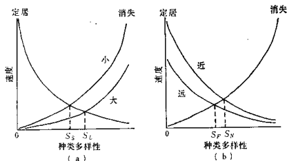
图2 在具有不同特征的岛屿上,种类多样性的定居和消失假说效应
