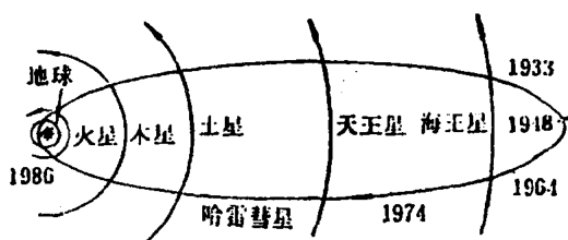
图1 哈雷彗星的轨道
