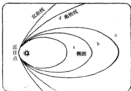
图2 三种轨道形式
