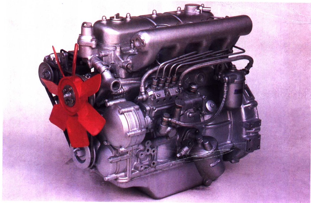
常柴牌N485Q柴油机
