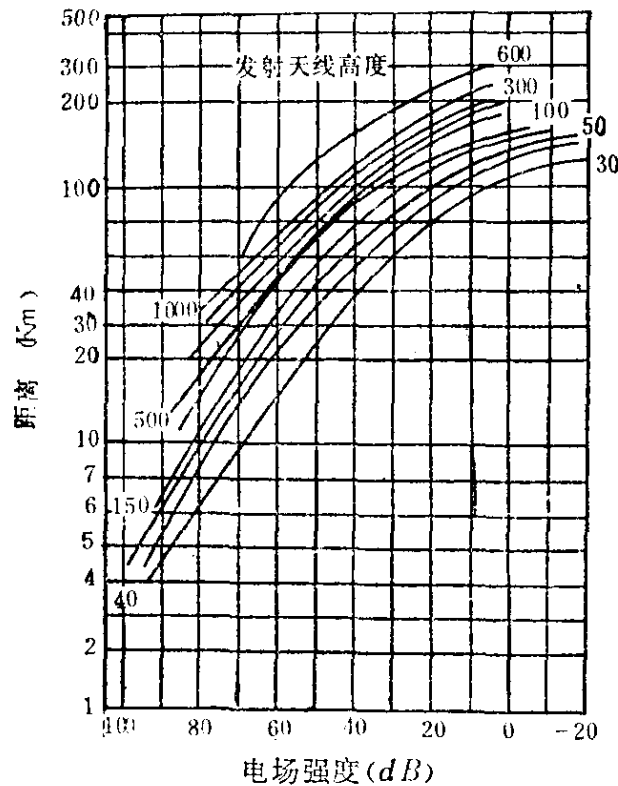
图 1—2 电场强度与传播距离的关系 ( P = 1 \text{ 千瓦} )
