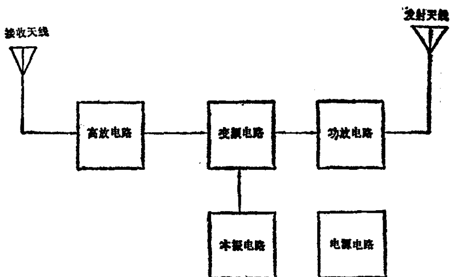
图 1—3 一次变频单通道电视差转机的组成
