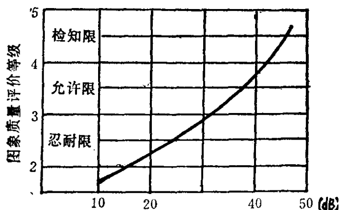
图1—1 图象质量评价与输出图象信噪比的关系
