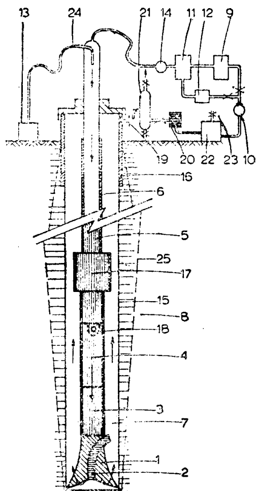
图 1.2 冷冻条件下钻井
