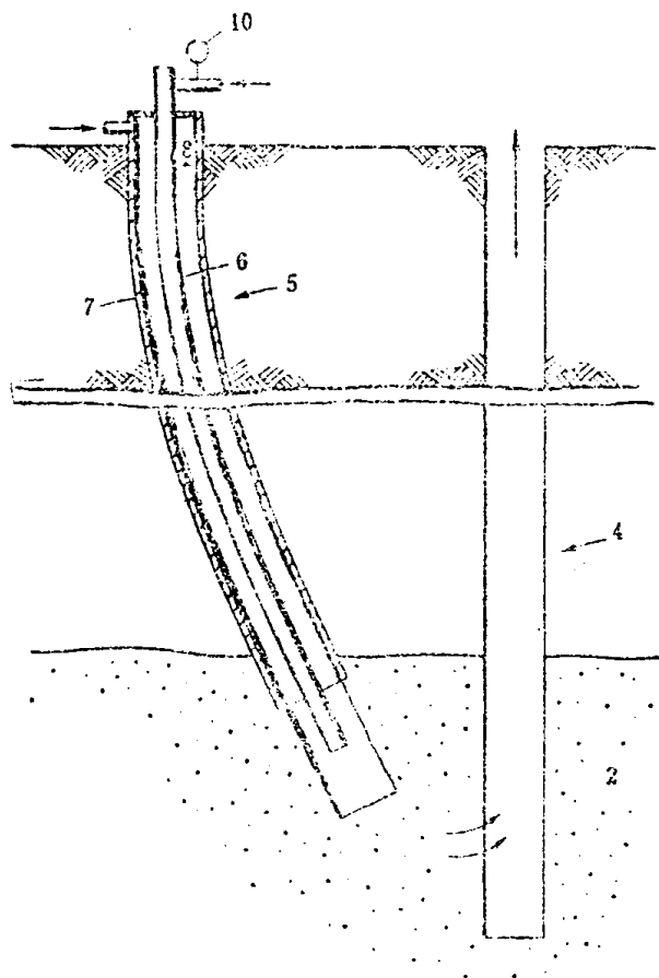
图 1.3 井喷事故井和救险井
