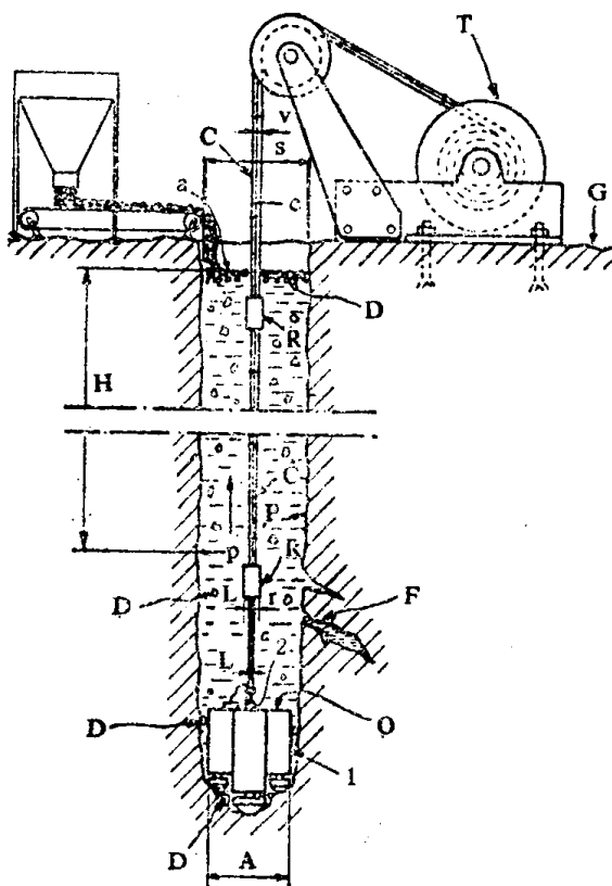
图 1.1 深井钻井设备
