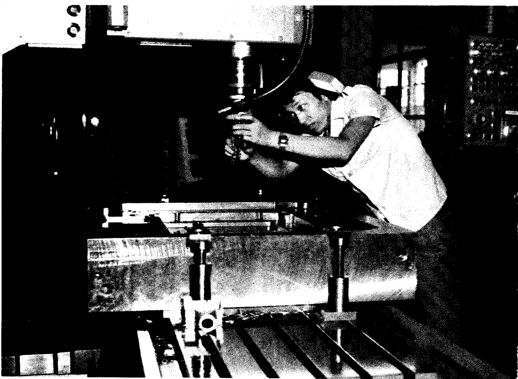
14 上海无线电十八厂使用大型数控仿形铣床，加快新品开发
