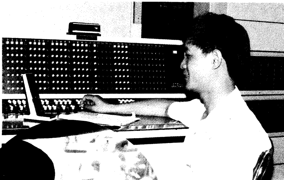
21 上海无线电二十四厂生产的转换台在长江航运局调度室运用
