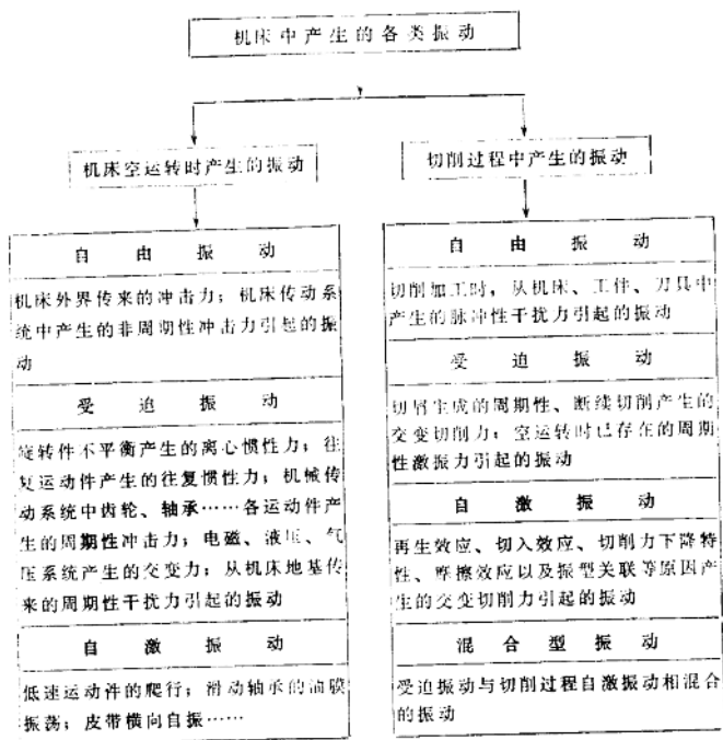
图1-2 机床振动的类型
