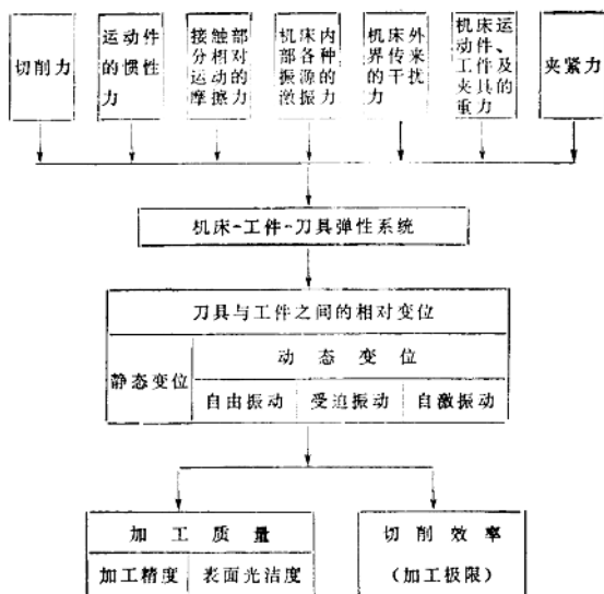
图1-1 作用在机床上的力及其影响
