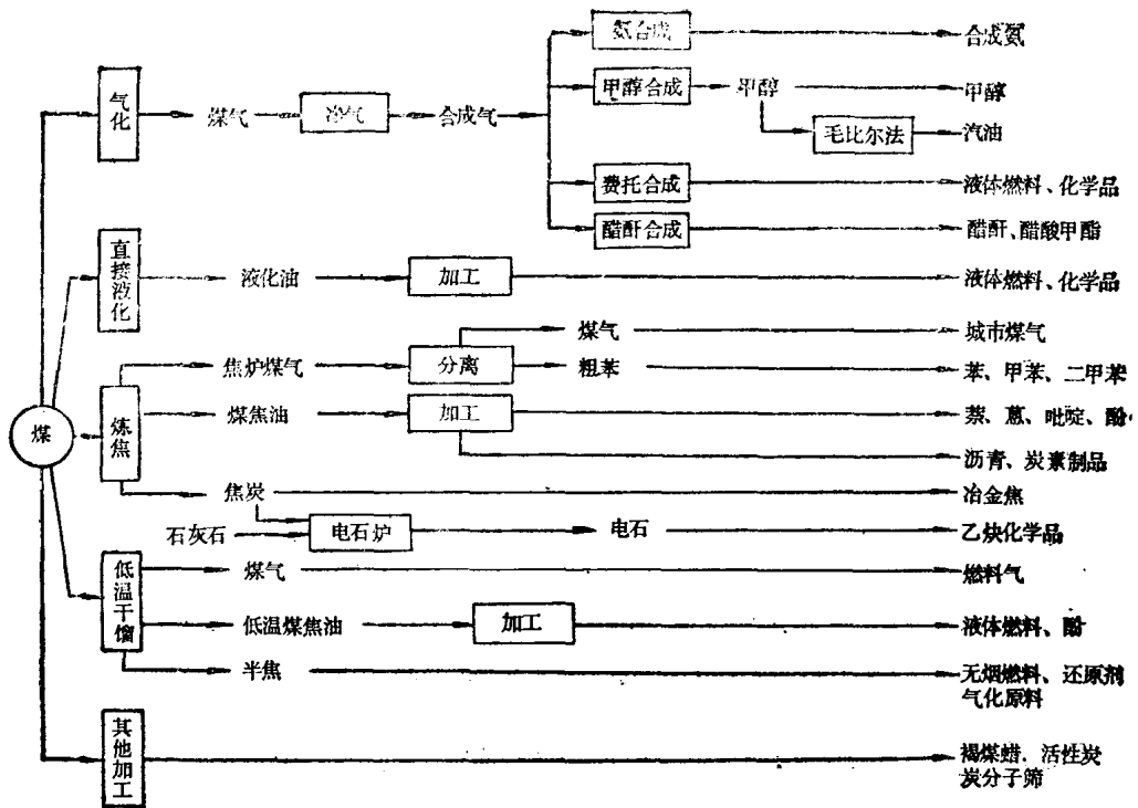
图 1-1 煤加工分类及产品示意图
