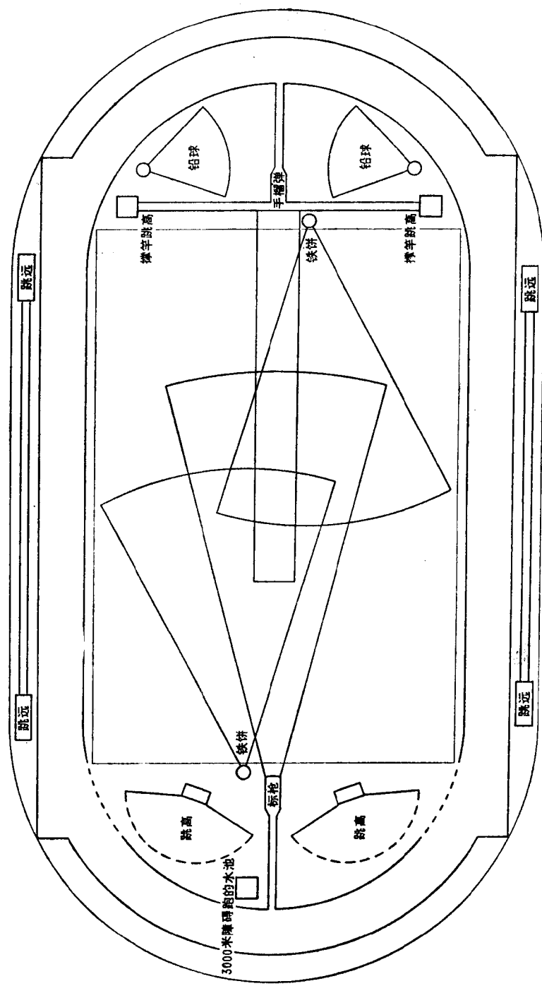
(一) 400米半圆式田径场上各项竞赛场地的分布图
