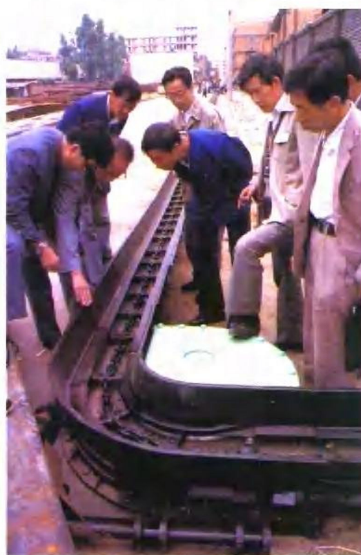
昆明煤矿机械总厂生产的可弯曲 90°刮板输送机
