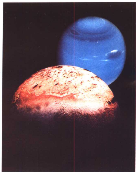
海王星及其卫星
