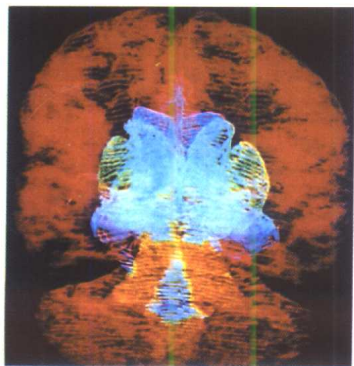
脑的后视图
