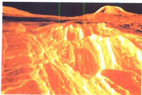
金星上面存在火山熔岩流
