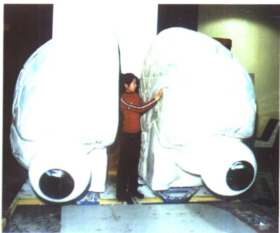
人脑的模型
