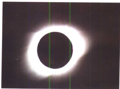
发生日全食时可见到壮丽的日冕
