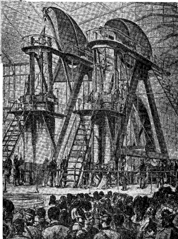
1876.5.10 费城万国博览会的开幕式，图中大机器即李圭所记之“哥阿力司”(Corliss)蒸汽机
