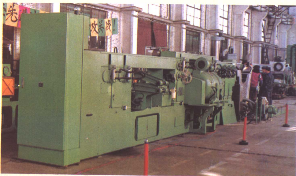
FB 101 型 晴纶直接制条机
