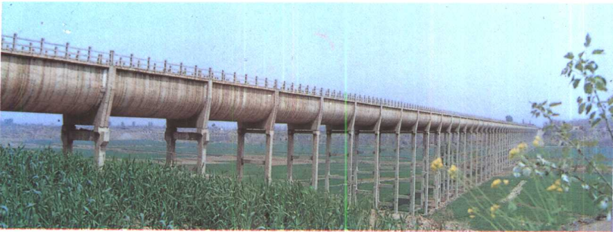
▲ 陆渾东一干渠马涧河渡槽
