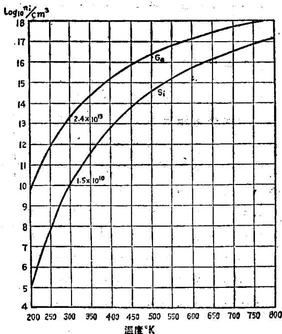
图 1-1-4 n_i 与温度的关系
