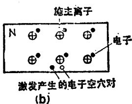
图 1-1-5 N型半导体
