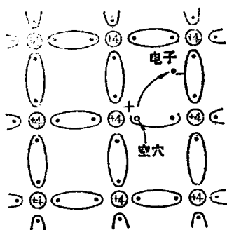
图 1-1-3 电子空穴对
