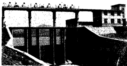
松树水库溢洪闸
