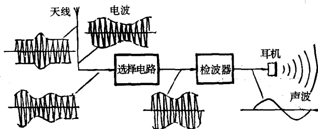
图 1-16 直接检波式收音机方框图
