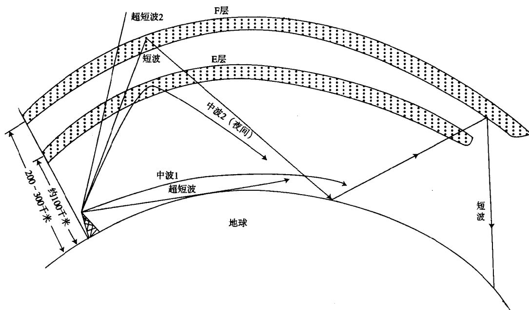
图 1-9 各波段无线电波的传播
