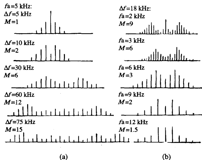
图 1-12 调幅信号与调频信号的频谱
