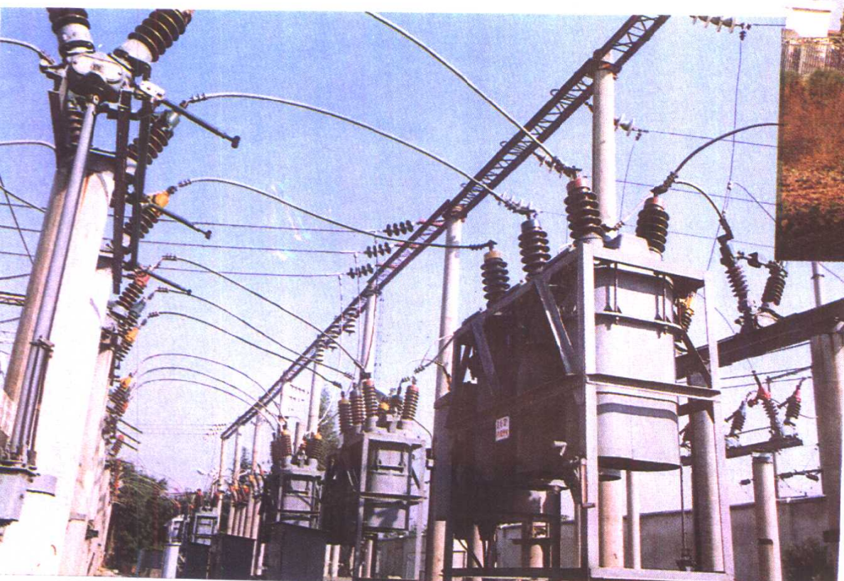
南陵县 110 千伏五里变电所
