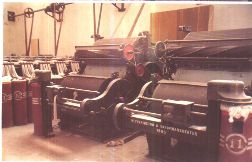
张謇从国外进口的纺织机械
