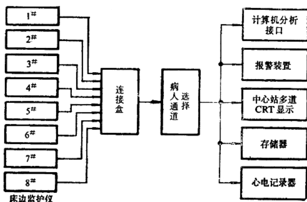
图 9-1 CCU 系统框图
