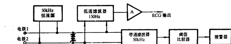
图 9-3 检测电极阻抗及电极脱落系统原理框图
