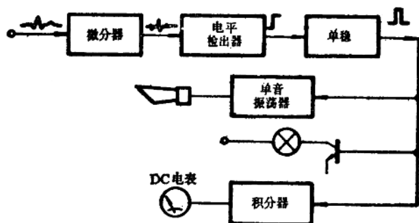
图9-6 积分模拟式平均心率计方框图
