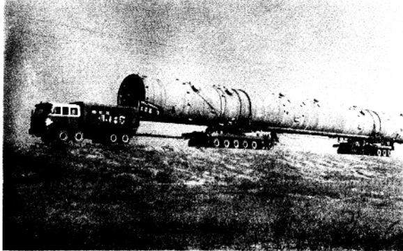
19. 我国自制的第一辆400吨大型公路平板车正运载着 长57米的超限大件设备 (沧州市交通局供稿)
