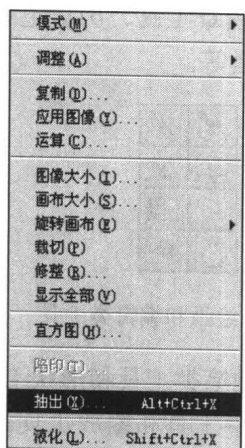
图 1.12 执行菜单项
