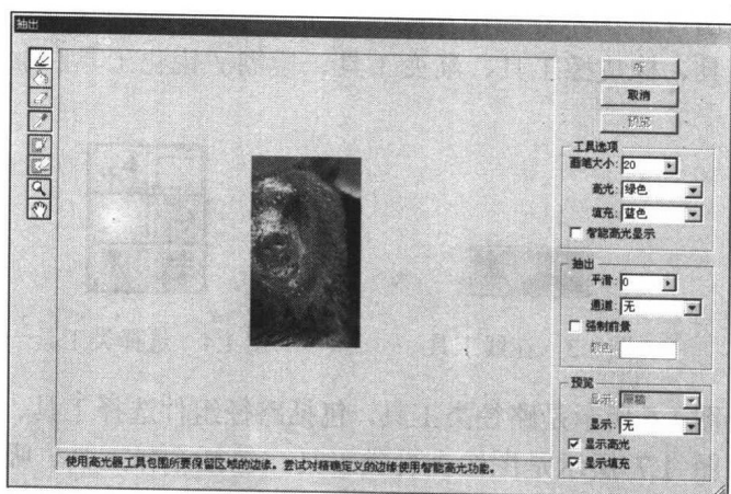
图 1.13 【抽出】对话框
