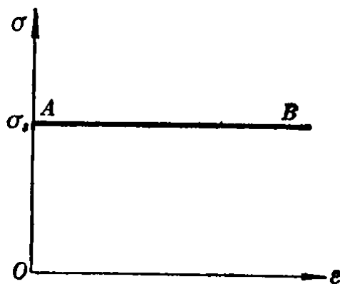
图 1-6 理想刚塑性模型
