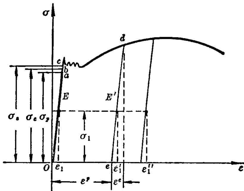
图 1-1 单向拉伸时的 \sigma - \epsilon 曲线
