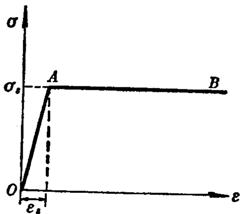
图 1-5 理想弹塑性模型
