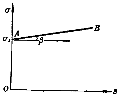
图 1-8 线性强化刚塑性模型
