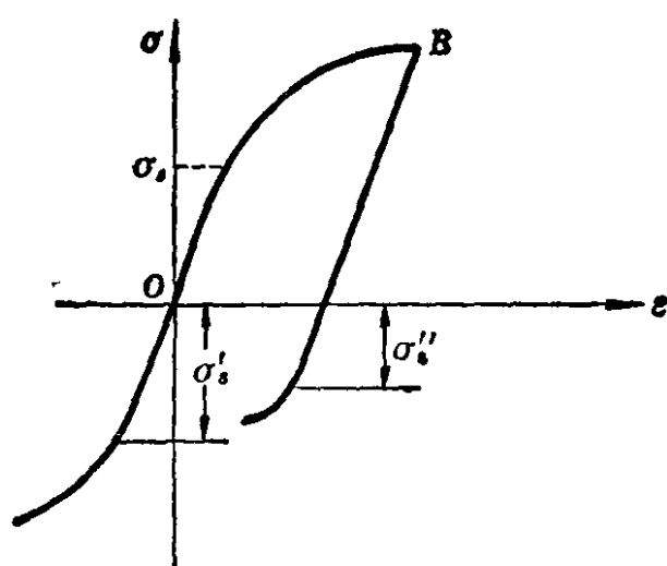
图 1-4 Bauschinger 效应
