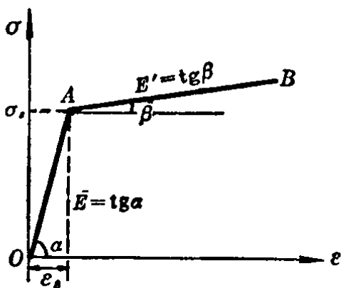
图 1-7 线性强化弹塑性模型
