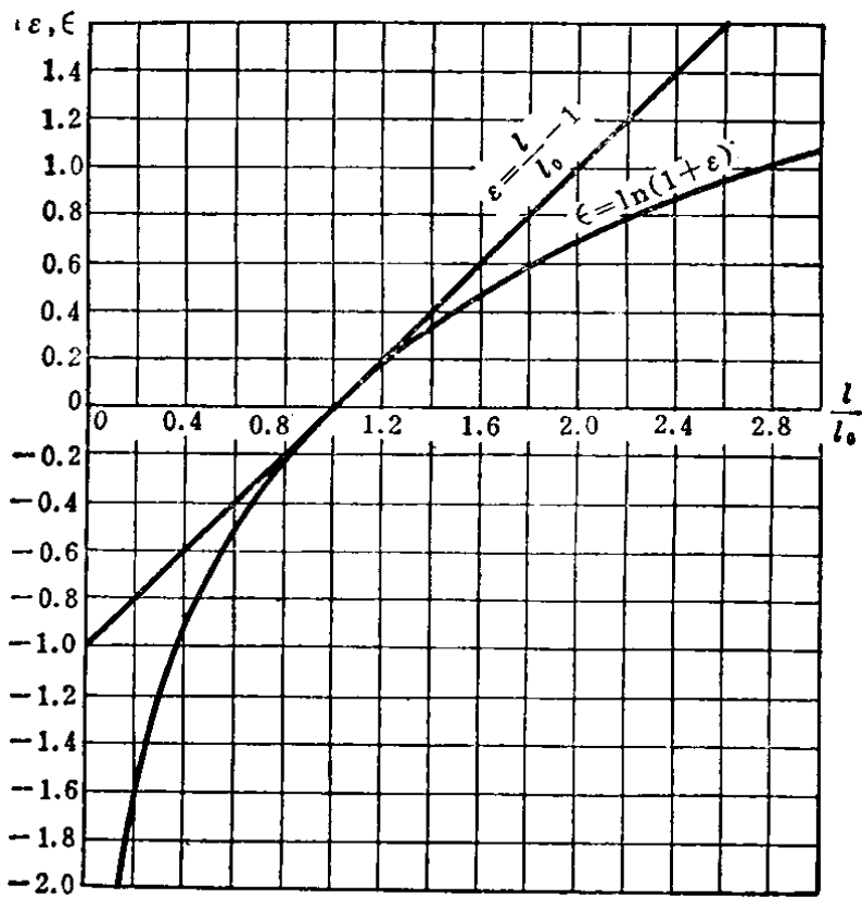
图 1-3 条件应变和对数应变
