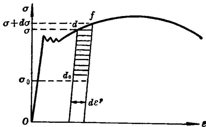
图 1-2 塑性功不可逆
