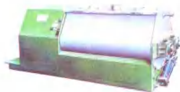
◁南京扬子粮 油食品机械厂生产的 WHJ200 型双 轴和面机
