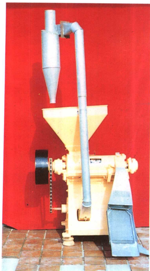
(16)县农机二厂 6NF—450 型 全分离式碾米机
