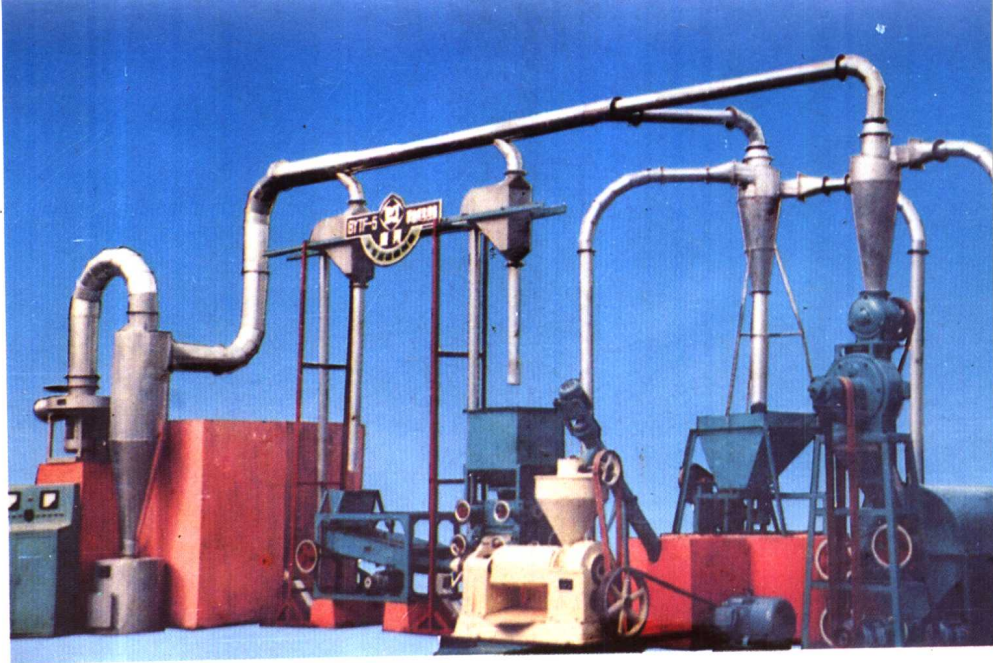
(15) 县农机一厂 6YFT—5 型榨油机成套设备
