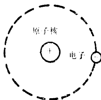
图 1-1 氢原子结构示意图
