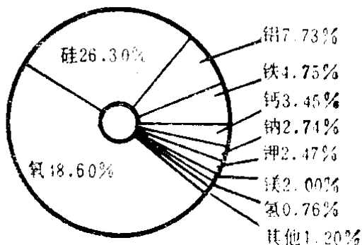
图 1-2 地壳中主要元素的百分含量
