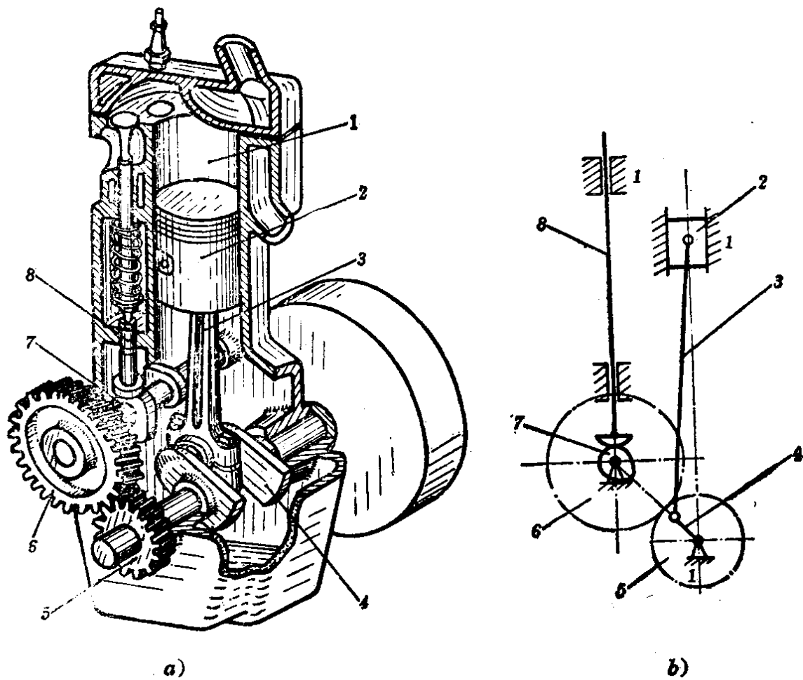
图 1-1 内燃机
