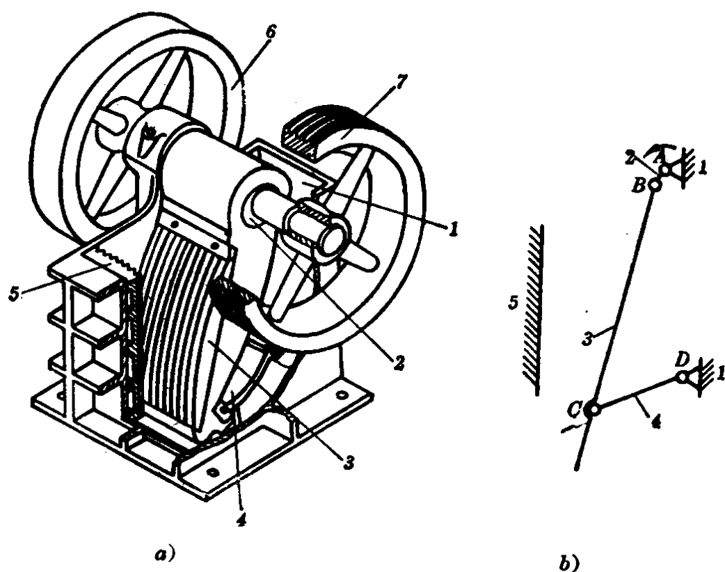
图 1-2 颚式破碎机
