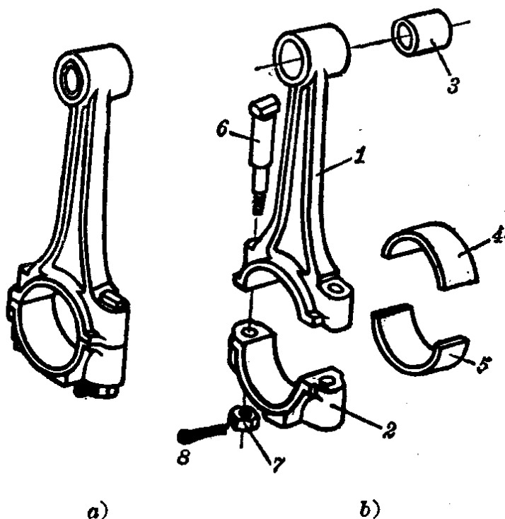
图 1-4 连杆
