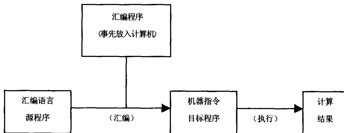
图 1.2 汇编过程
