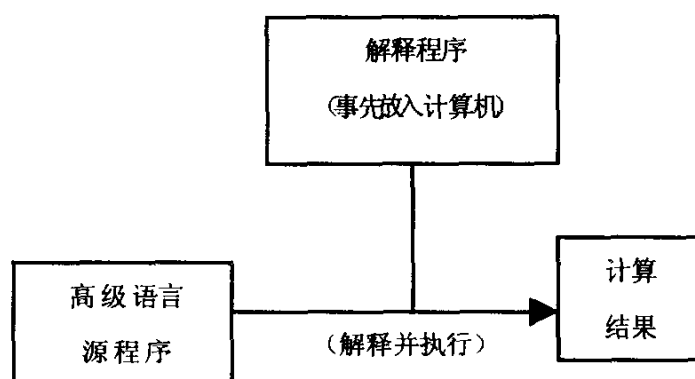
b)解释过程
