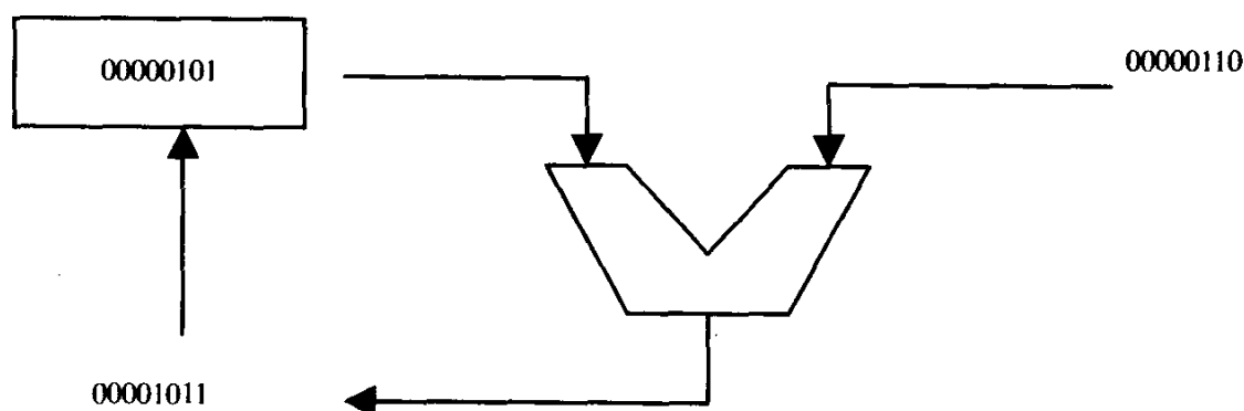
图 1.1 执行过程
