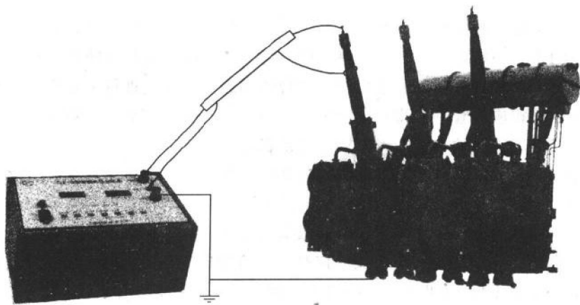
图 1-1 试品绝缘电阻测量示意图
