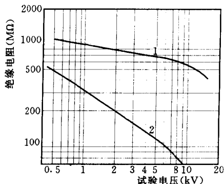
图 1-4 某试品绝缘电阻—电压特性曲线 1—绝缘合格；2—绝缘受潮或老化
