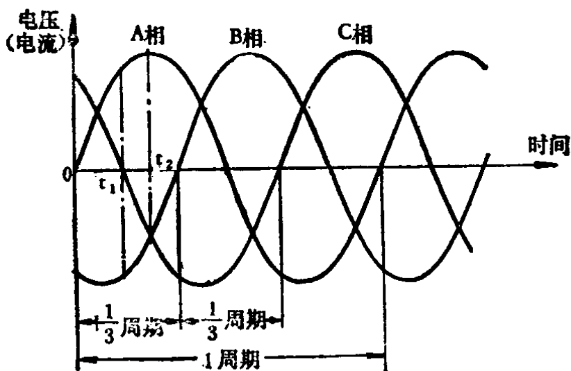
图6 三相交流电的正弦曲线
