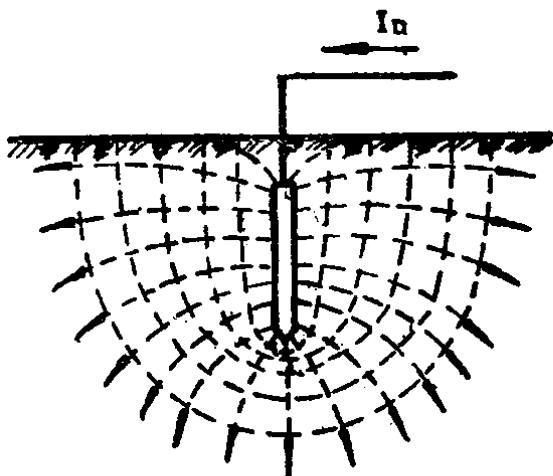
图 8 地中电流呈半球形流散
