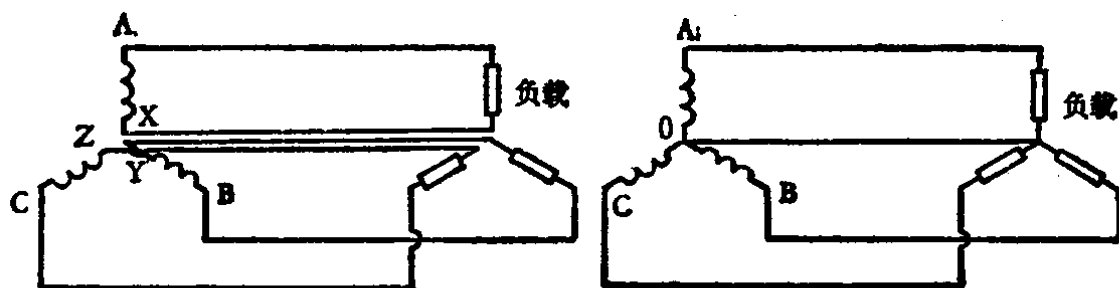
图5 三相交流电的星形接法
