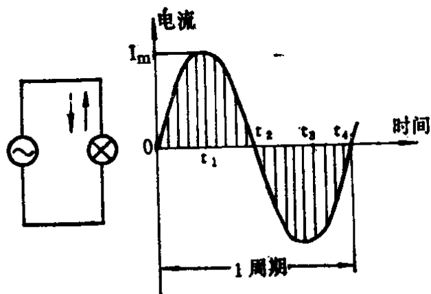
图 4 交流电的正弦曲线
