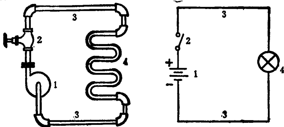
图1 水路和电路的比较
