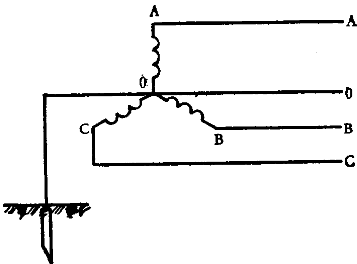
图 7 火线、零线示意图
