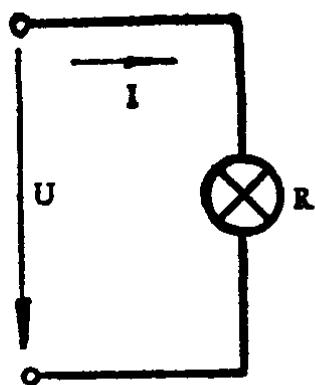
图2 欧姆定律示意图
