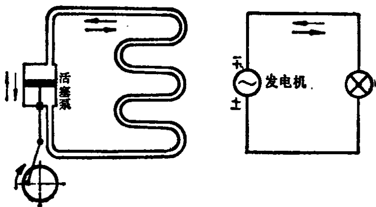
图3 水路和交流电路的比较
