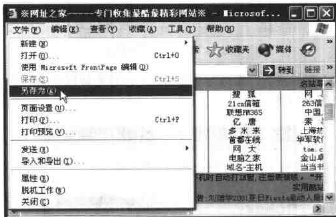
图 1-10 另存为窗口
